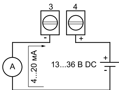
Рисунок 3 — Подключение датчика
