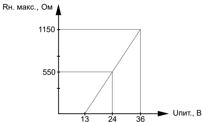
Рисунок 1 — Максимально допустимая нагрузка на выходе датчика
