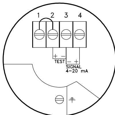
Рисунок 2 — Клеммник датчика
