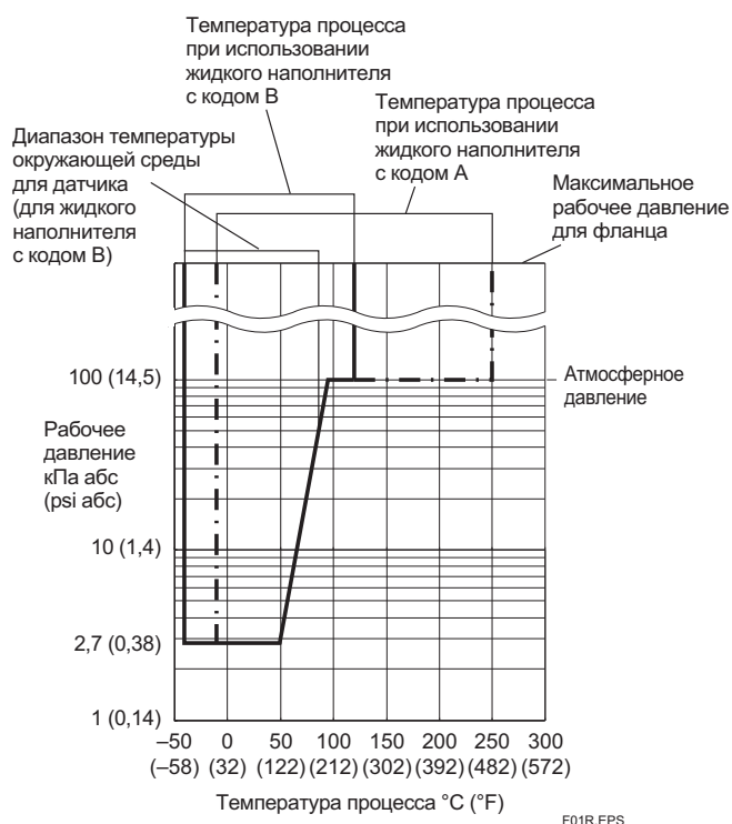
Рис. 1. Рабочее давление и температура процесса (Жидкий наполнитель: силиконовое масло для общего и высокотемпературного применения)
